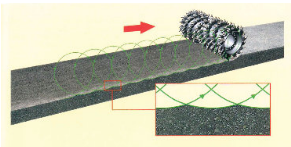
Einfluss der Fräsgeschwindigkeit auf die Oberflächentextur
